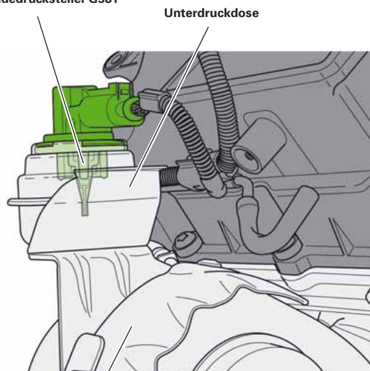
Positionsgeber für Ladedrucksteller G581
