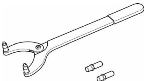
T10172 Gegenhalter
