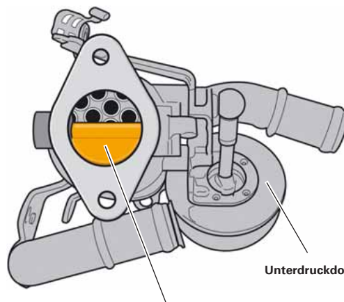
Abgaskühlung aktiv
