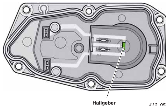
Deckel Abgasrückführungsventil
