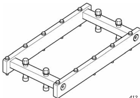
T10262 Rahmen
