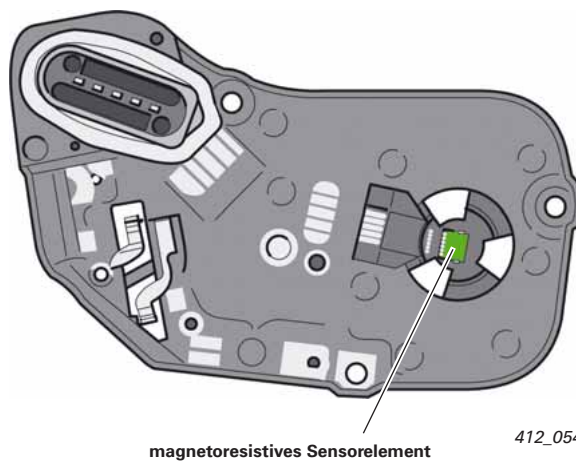
Schaltplatine
