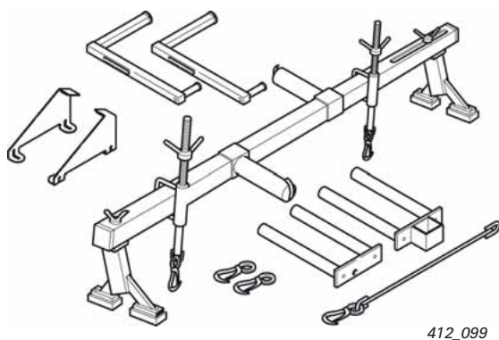
10-222A Abfangvorrichtung
