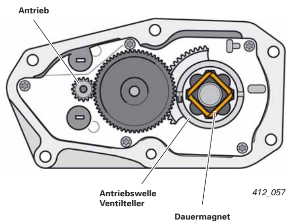
Gehäuse Abgasrückführungsventil
