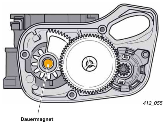
Gehäuse Saugrohrklappe
